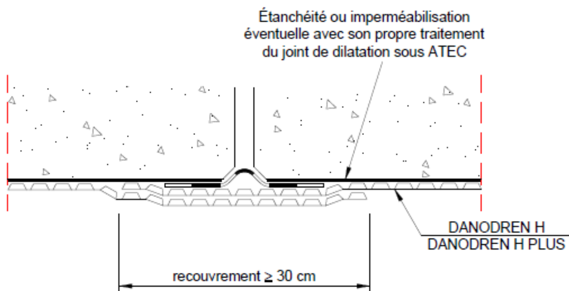
Figure 8 - Joint de dilatation - zones de sismicité conduisant à des déplacements inférieurs à 2 cm
