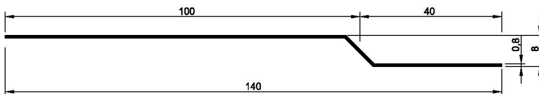
Figure 3 bis - Moulure DANODREN Protection (acier galvanisé)
