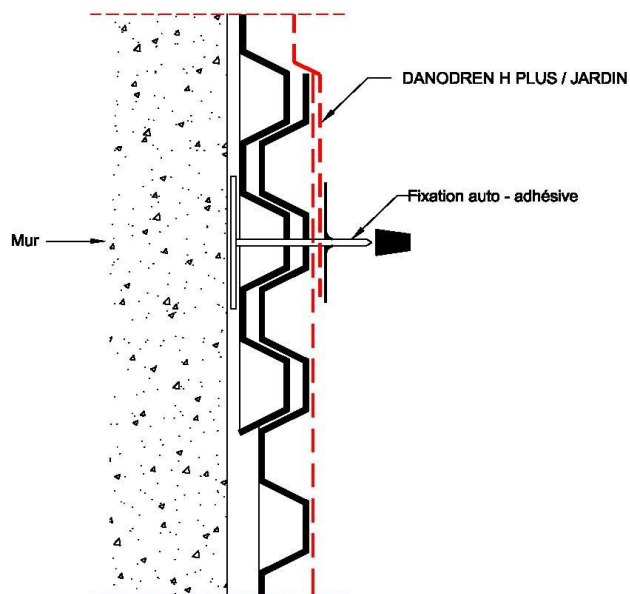
Figure 4 bis - Fixation haute de la nappe DANODREN H15 PLUS, DANODREN H25 PLUS et DANODREN Jardin – Support maçonnerie
