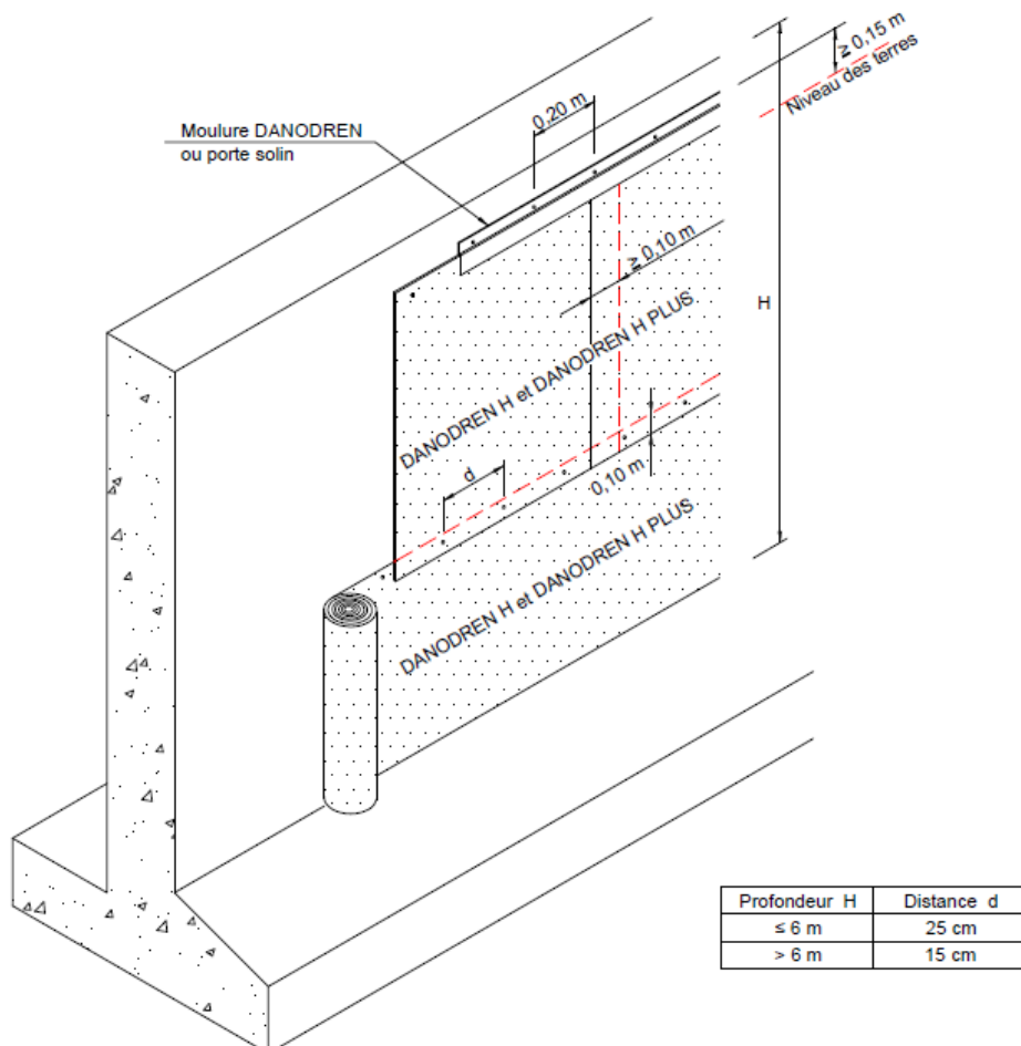
Figure 6 ter - Schéma de principe sans revêtement d'étanchéité (sens de pose horizontal)
