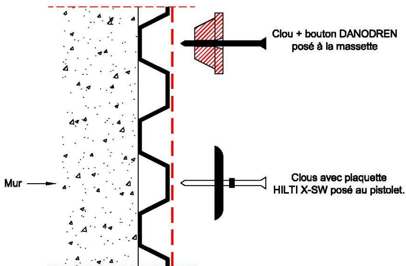
Figure 4 bis - Fixation haute de la nappe DANODREN H15 PLUS, DANODREN H25 PLUS et DANODREN Jardin – Support maçonnerie
