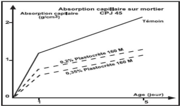
Evolution de l'absorption capillaire sur éprouvettes à 7 jours d'âge (Selon NF P 18-354)
